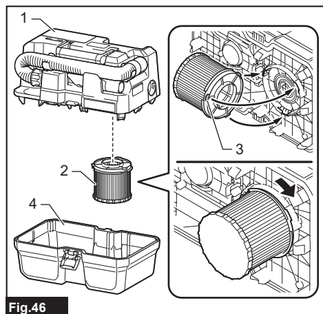
► 1. Tête 2. Filtre HEPA 3. Rebord de fixation 4. Réservoir
